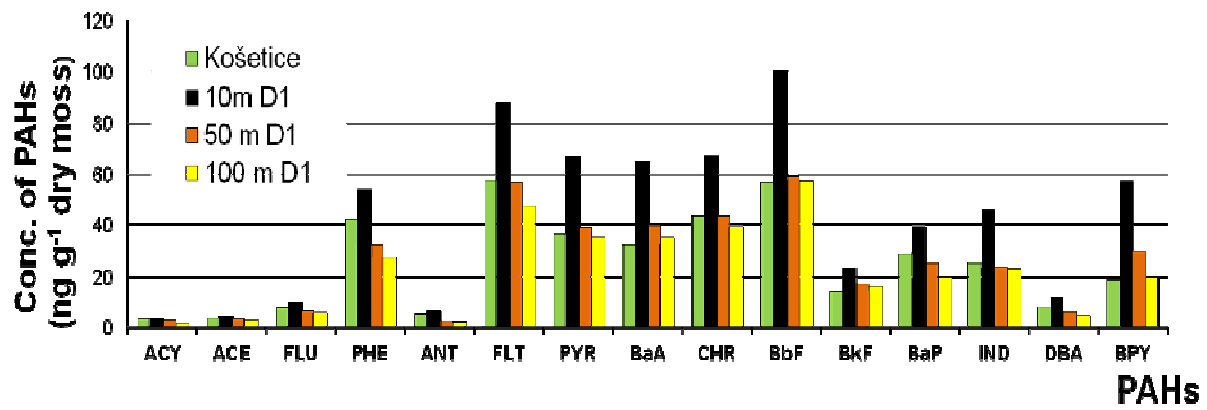
Obr. 7 Koncentrace vybraných polycyklických uhlovodíků v mechu do vzdálenosti 100 m od dálnice D1 (km 39) a v lese u Košetice.
