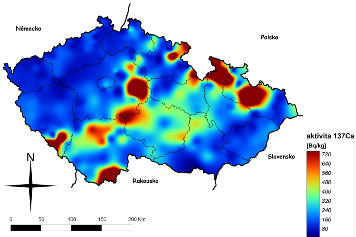
Obr. 9 Obsah ^{137}\text{Cs} v lesním nadložním humusu na území ČR v roce 2005.
